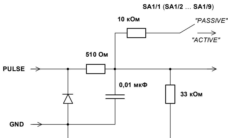
Рис.В.1. Схема входного каскада импульсных входов.
